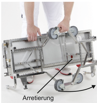
1a. Bein arretierung am Rahmen lösen und rechtes Bein ausklappen.
