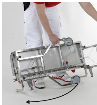
1c. Linkes Bein ausklappen.
