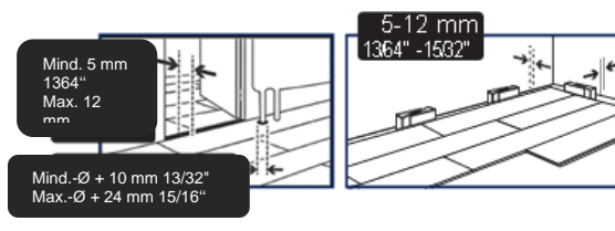
DEHNUNGSFUGE
