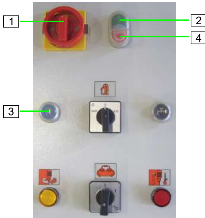
Abb. 78: Rückwärtslauf
