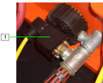
Abb. 87: Druckschalter Wasser
