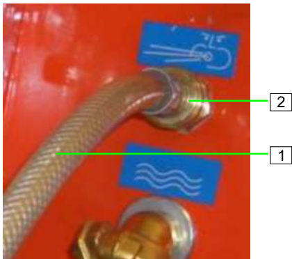
Abb. 39: Luftschauch anschließen
