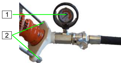
Abb. 79: Mörteldruck überprüfen und ablassen
