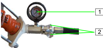
Abb. 64: Mörtelschlauch abkuppeln
