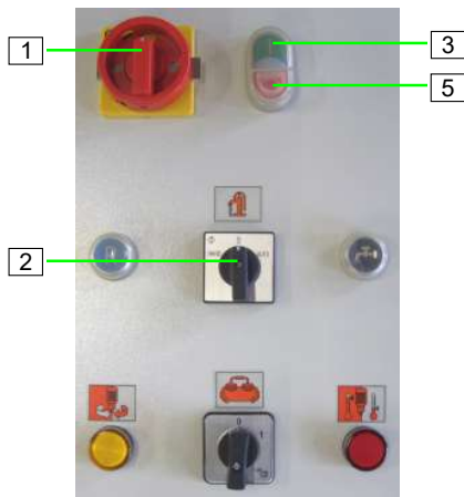
Abb. 46: Maschine einschalten
