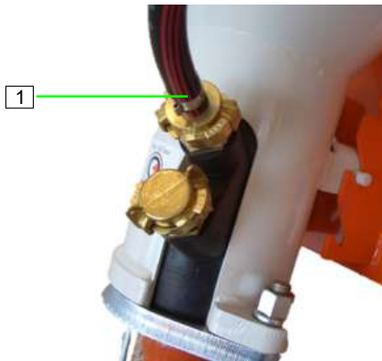
Abb. 67: Wasserschlauch anschließen
