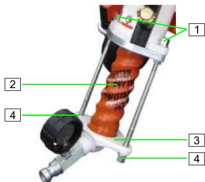
Abb. 73: Pumpeneinheit abnehmen
