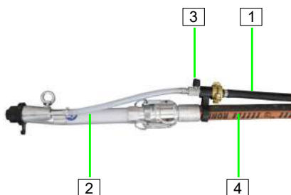
Abb. 40: Spritzgerät
