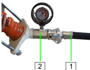
Abb. 37: Mörtelschlauch anschließen
