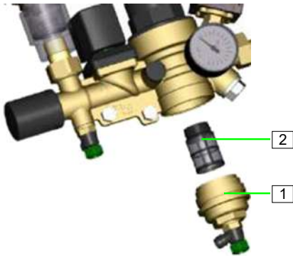
Abb. 28: Schmutzfängersieb prüfen
