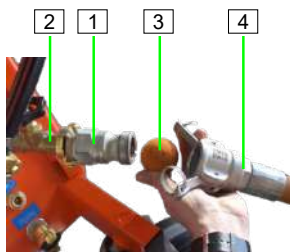
Abb. 65: Mörtelschlauch reinigen
