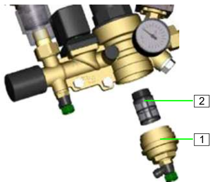
Abb. 86: Schmutzfängersieb
