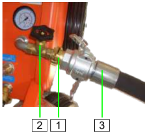
Abb. 36: Mörtelschlauch vorbereiten
