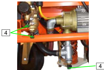
Abb. 60: Ablasshähne öffnen
