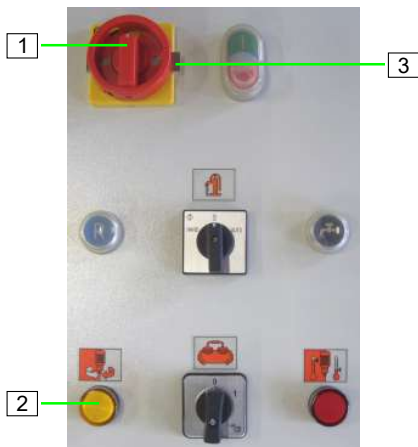
Abb. 32: Maschine einschalten
