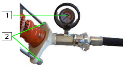
Abb. 57: Mörteldruck überprüfen und ablassen
