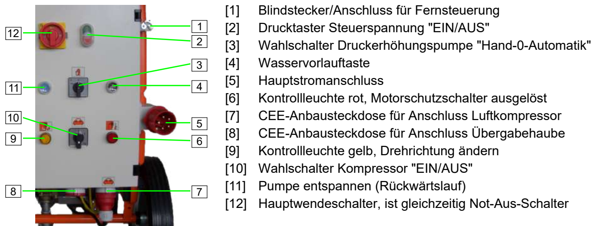
Abb. 14: Baugruppe Schaltschrank
