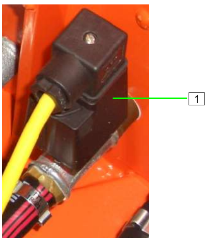
Abb. 88: Druckschalter Luft
