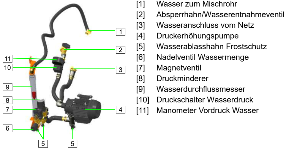
Abb. 15: Baugruppe Wasserarmatur
