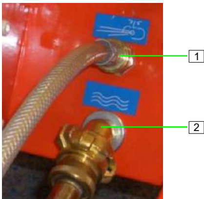
Abb. 61: Luftschlauch anschließen
