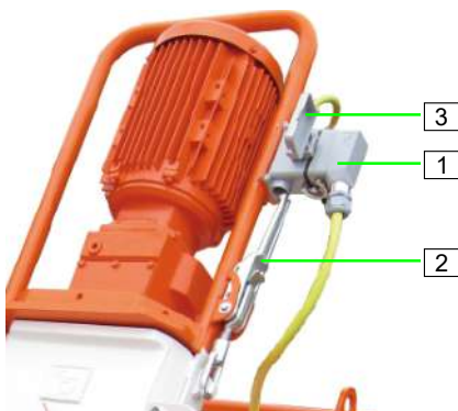
Abb. 68: Motorkippflansch öffnen
