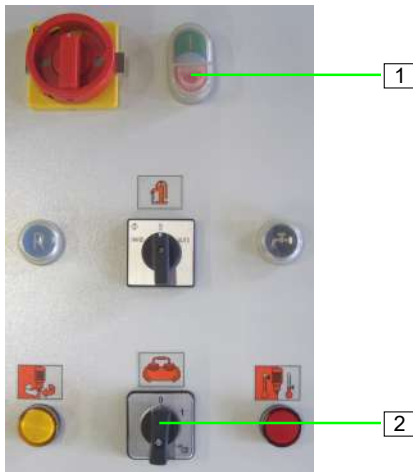
Abb. 63: Arbeitsende
