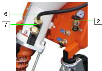
Abb. 34: Wasserentnahmeventil
